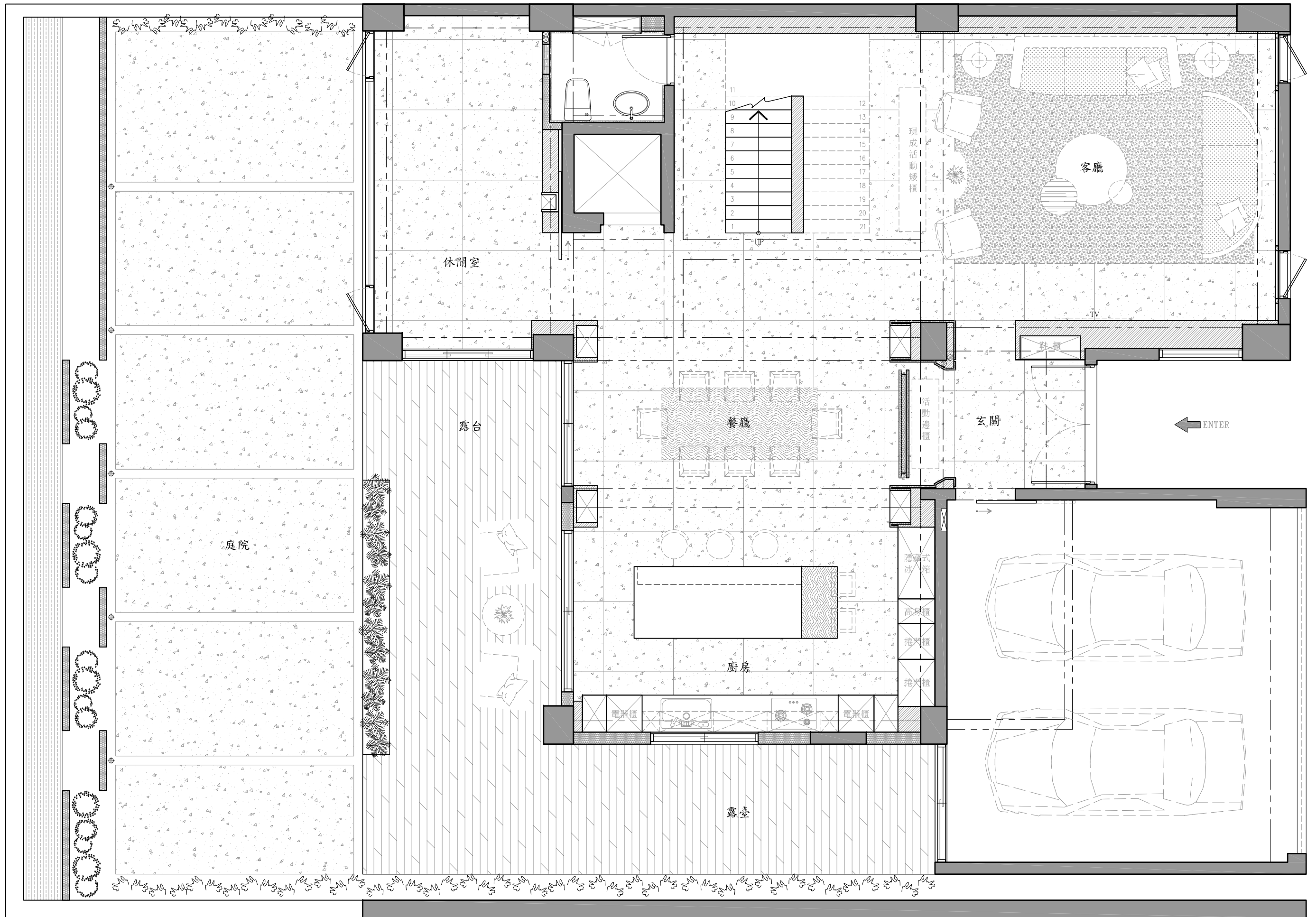
山漸青透天別墅A42 一樓平面配置圖
